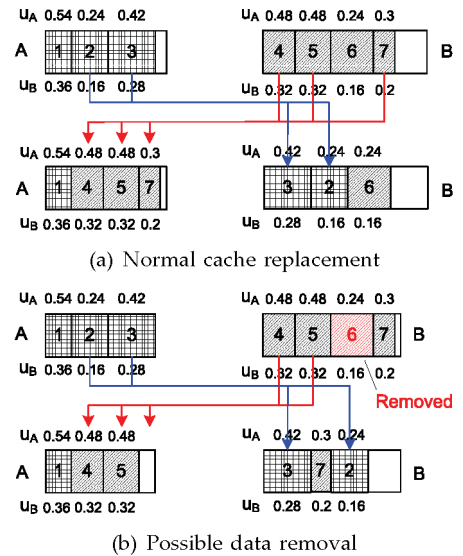
Fig. 10. Cache replacement.
